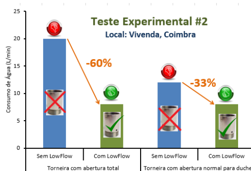
Fig. 8. Poupança de água obtida em moradia.
